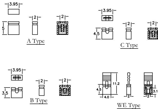
2106-Series 2.0mm(0.079")
